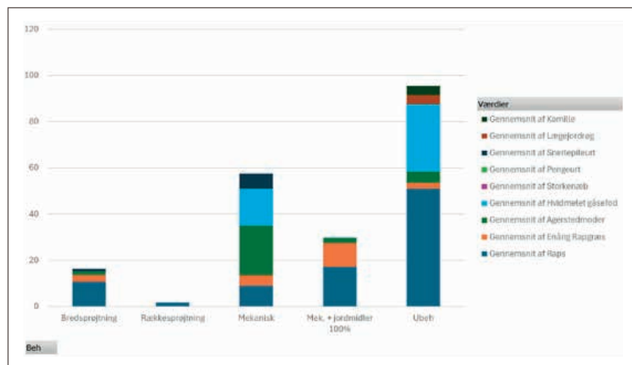
Figur 1. Ukrudtsdække i procent, Sukkerroer ved Ødemark Gods, 10. juni 2025.
