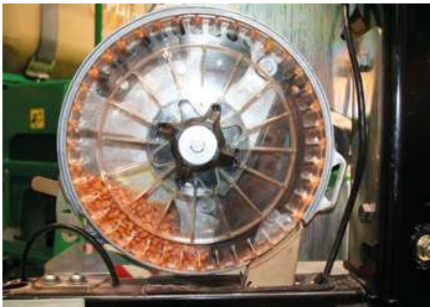
Billede 1: Sånhed til majs fra Great Plains, der viser vacuum-teknik i en moderne enkorns-såmaskine. Foto: Otto Nielsen, NBR
